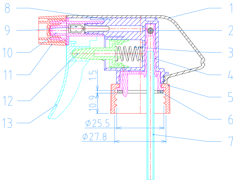
(28/400W) CAP , P=1"x8 TPI
