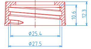
(28/400) CAP, P=1"x8 TPI
